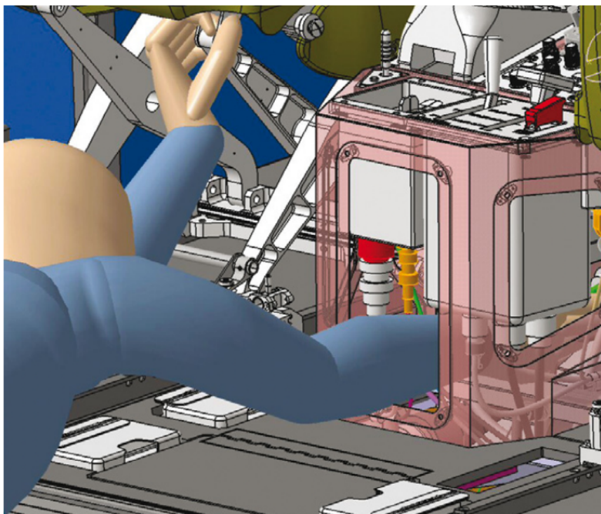
Validation d'une opération de production par simulation dans Delmia de l'éditeur Dassault Systèmes.
